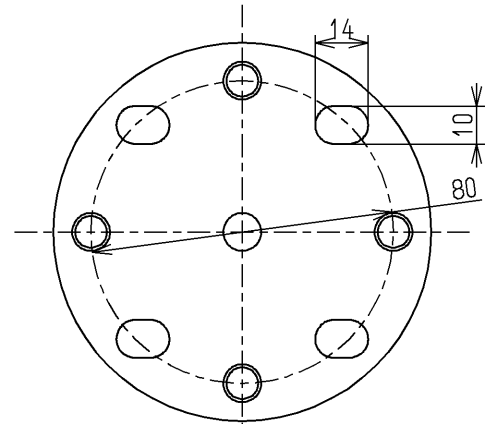
取付座詳細(1:2)
