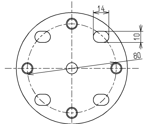
取付座詳細(1:2)
