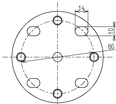
取付座詳細(1:2)
