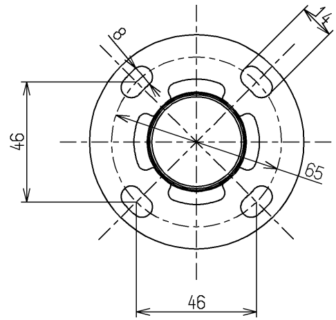
取付座詳細(1:2)
