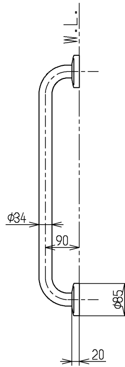
取付座詳細(1:2)
