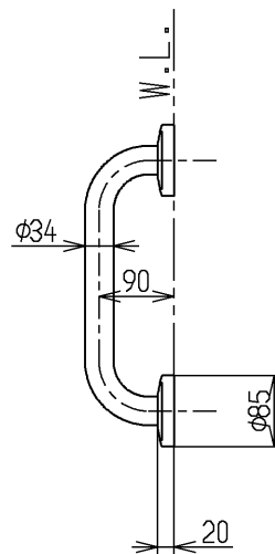
取付座詳細(1:2)
