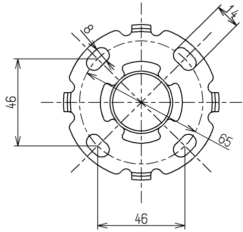
取付座詳細(1:2)
