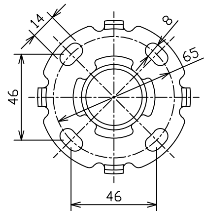
取付座詳細(1:2)
